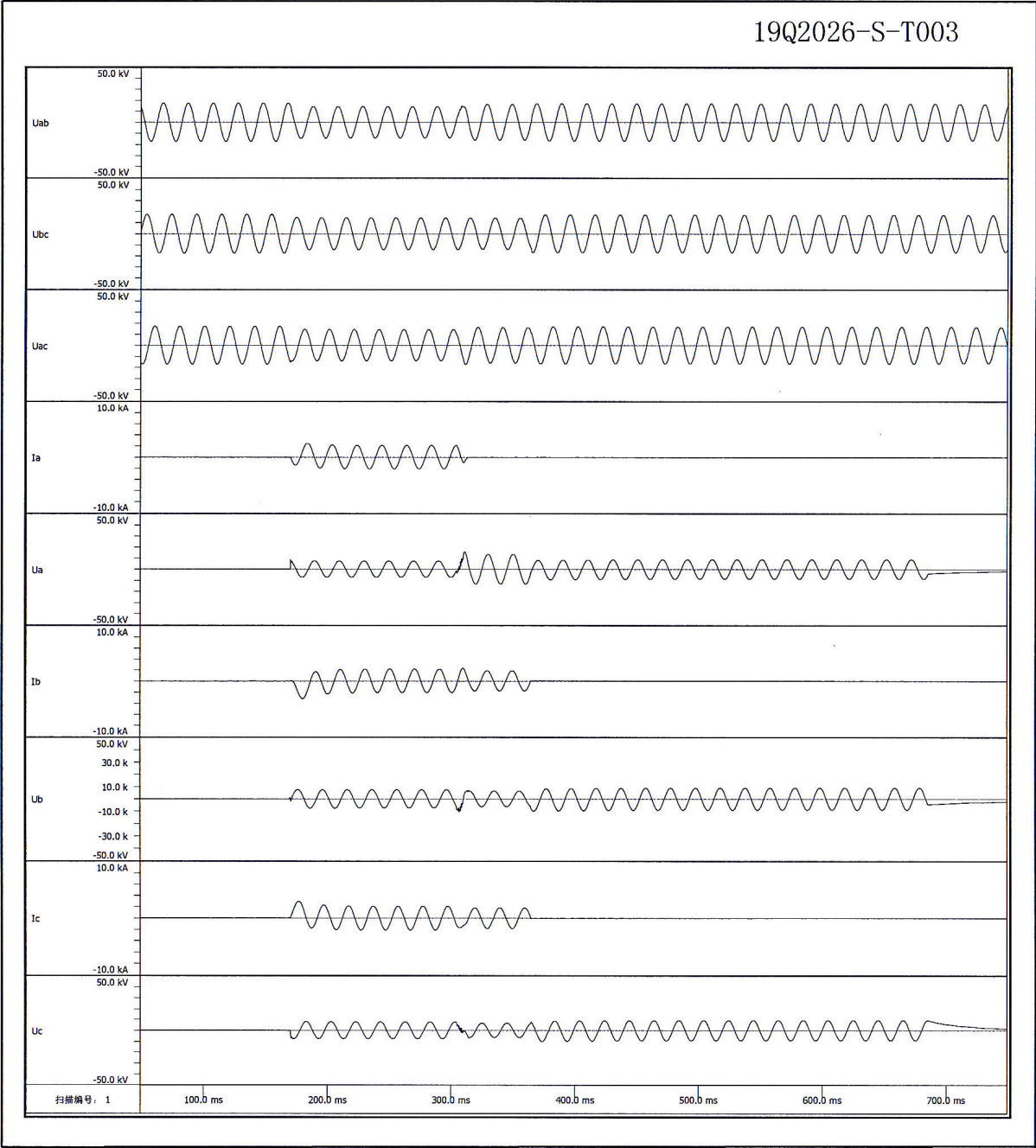
示 波 图
