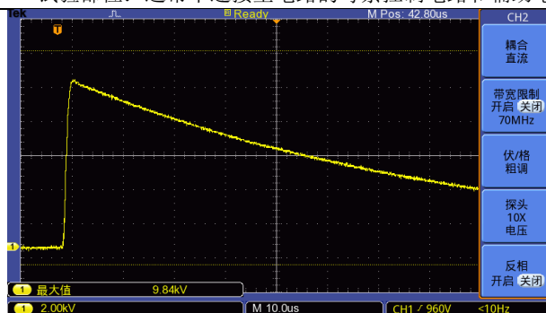
冲击耐受电压试验示波图 (9.8kV)
